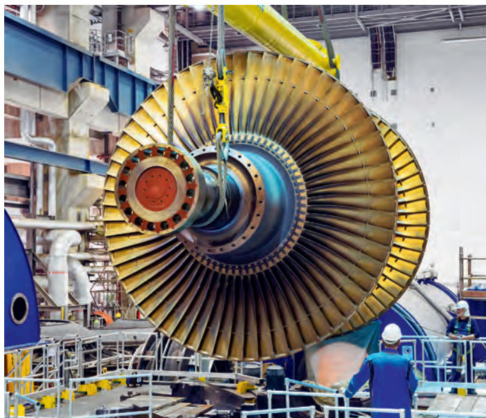
↑ SCHWERSTARBEIT: Für die Revision müssen die Turbinen aus ihrem Lager gehoben werden.
