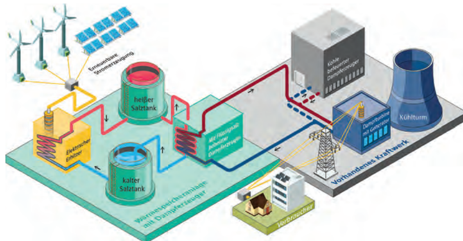
↑ SMARTE Lösung: Der überschüssige Strom aus Wind- und Solarkraft erhitzt Flüssigsalz in den Wärmespeichern. Die Hitze nutzt das Kraftwerk bei Strombedarf zum Antrieb der Turbinen.
